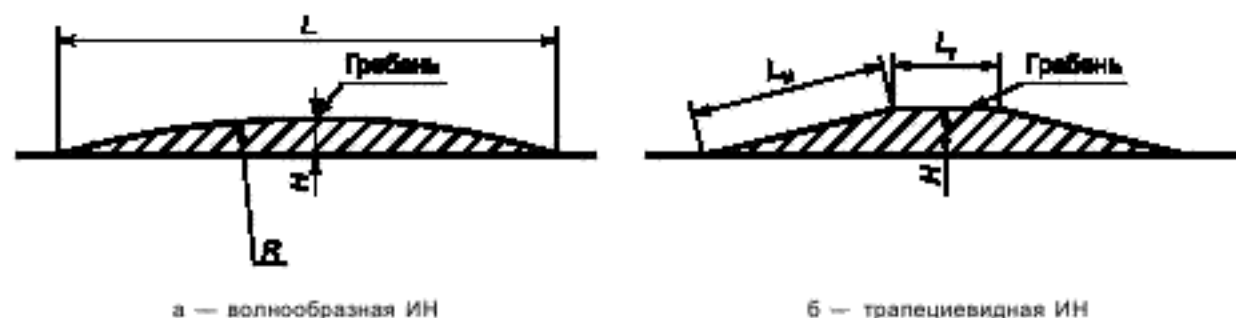
Рисунок 1 — Поперечные профили ИН
