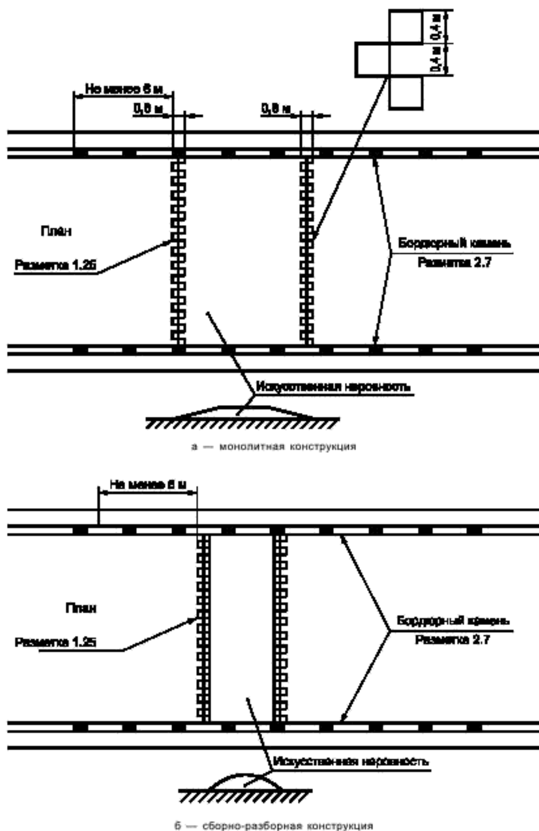
Рисунок 4 — Пример нанесения разметки 1.25 и 2.7 при устройстве ИИ
