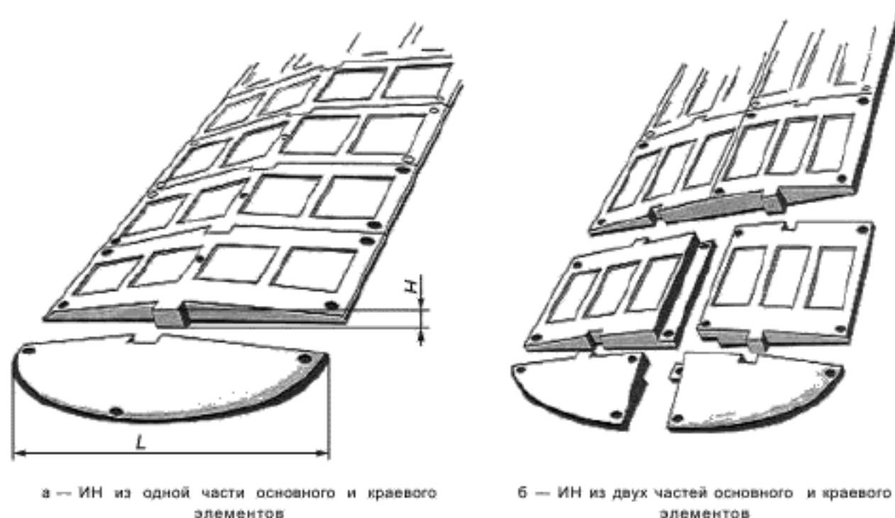
Рисунок 3 — Конструкция сборно-разборной ИН
