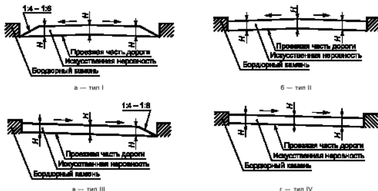
Рисунок 2 — Продольные профили ИН
